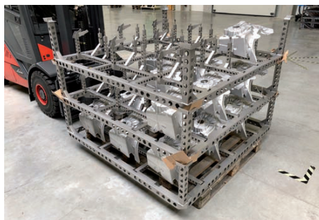
Das Warenträger-System besteht aus einer wiederverwendbaren Grundträgerkonstruktion und einer spezifischen Bauteilaufnahme
